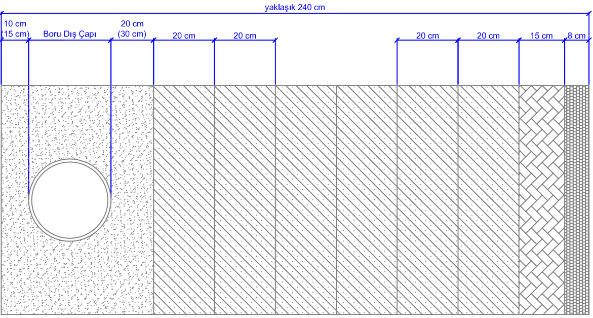
KANALİZASYON ANA HAT Ø200-400 (Ø400'den büyük) BORULARI İÇİN ASFALTA DOLGU DETAYI
